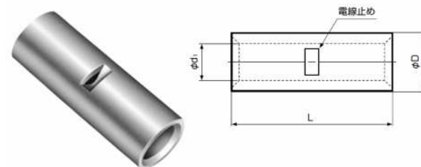
突き合わせ用スリーブ（B形）
