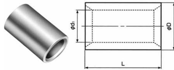
重ね合わせ用スリーブ（P形）
