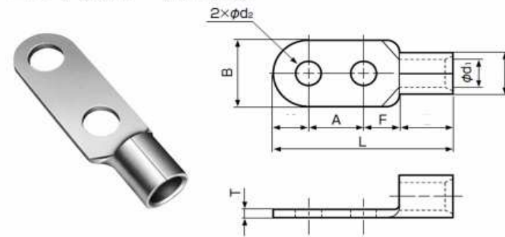
ニツ穴端子（RD形）
